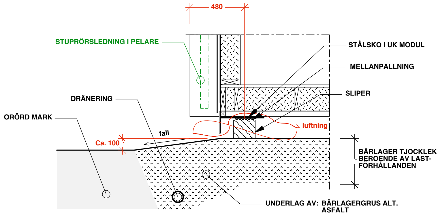
SEKTION A SKALA 1:20
